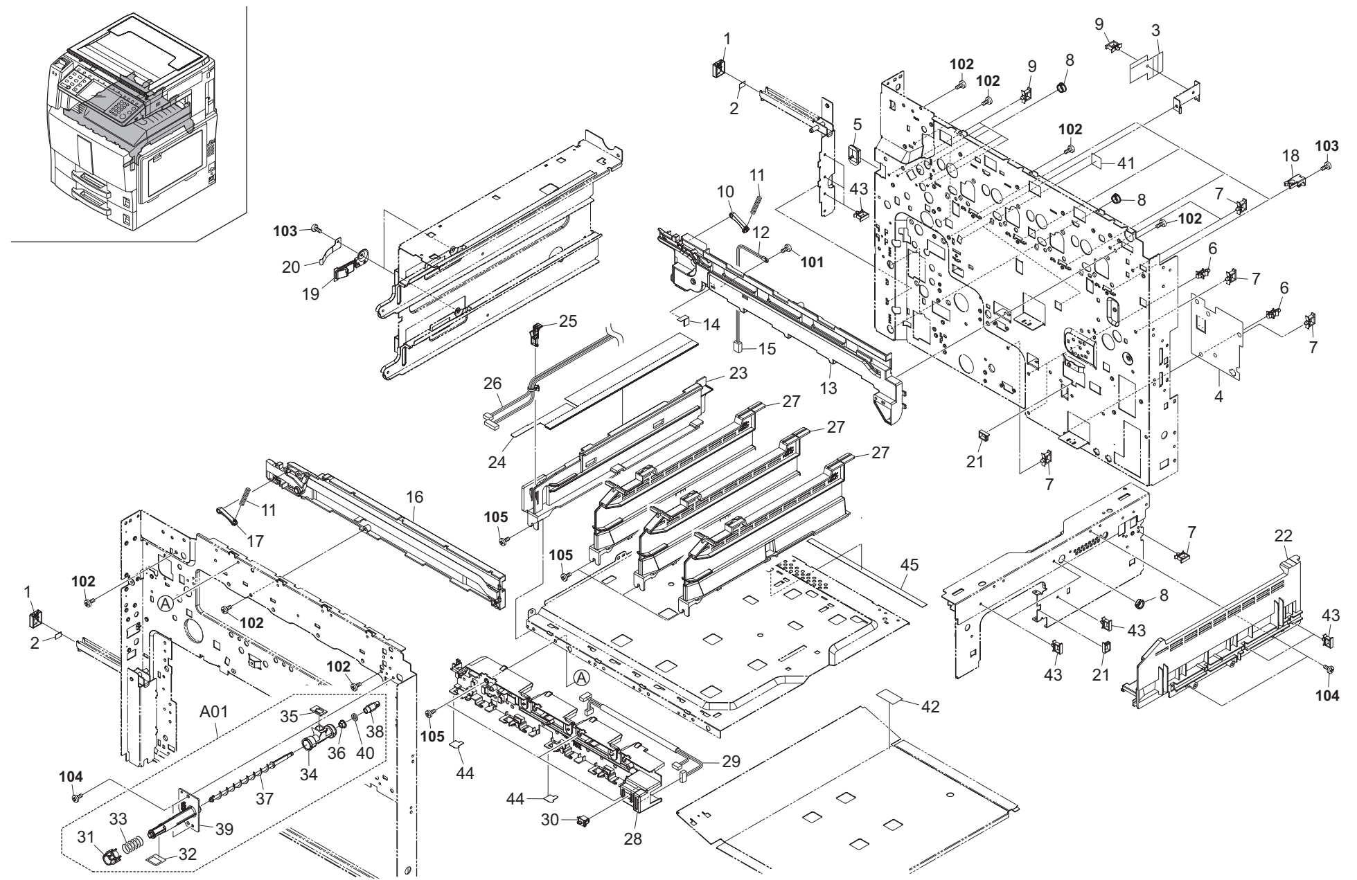
FIG. 3 Frames 1
